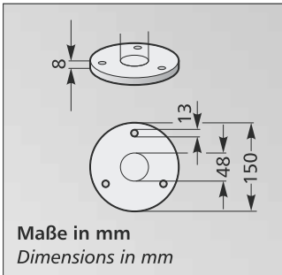
Fußplatte zum Aufdübeln. Base plate for bolting.
